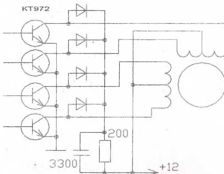
Рис. 4. Электрическая схема драйвера.
