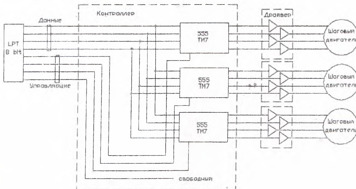
Рис. 2. Структурно – функциональная схема системы управления ШД.
